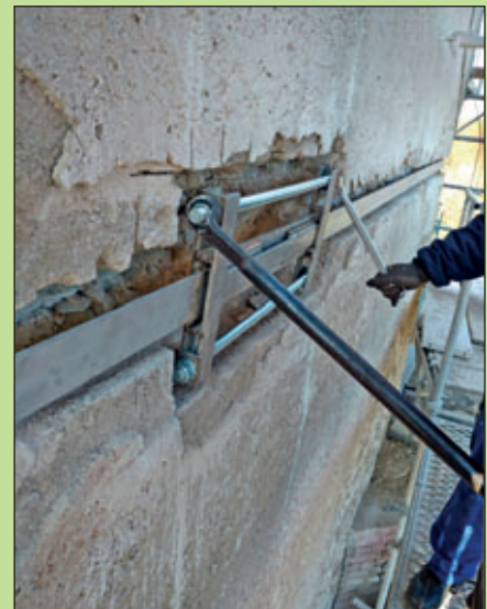
Vorspannen der Stahlgurte um den Turm
